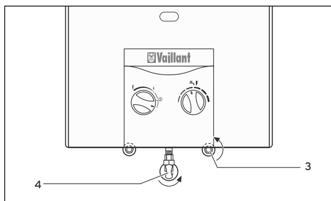
Fig. 4.2 Dispositivos de bloqueo, tipo (X)F
