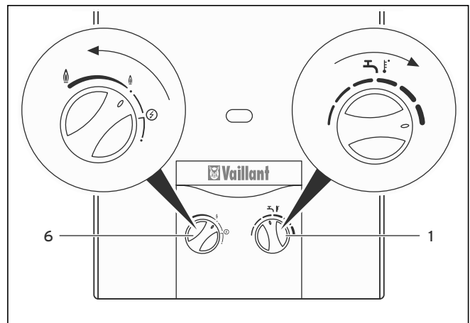
Fig. 6.2 Ajuste de temperatura y potencia máximas, tipo (X)F
